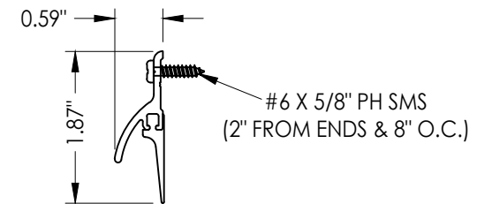
11 DOOR BOTTOM SWEEP
