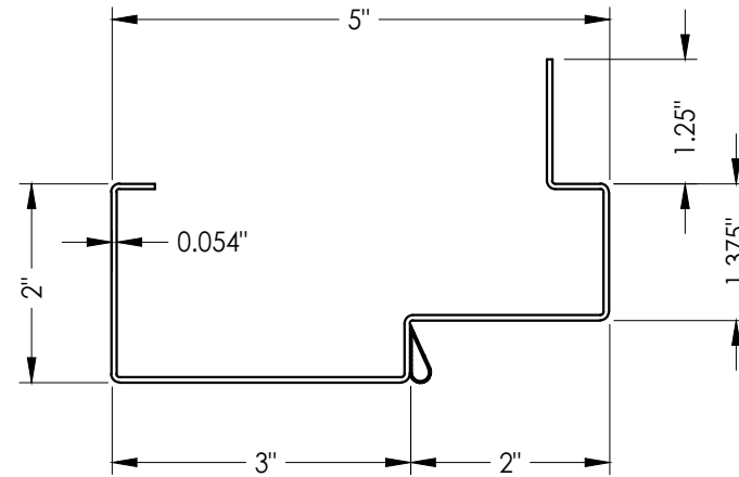
1 HOLLOW METAL FLANGE FRAME 16 GA.
